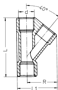
Разделительные фитинги серия EYS 1 ... 3
