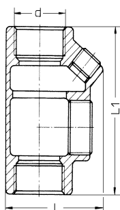
Разделительные фитинги серия EYS 5 ... 8
